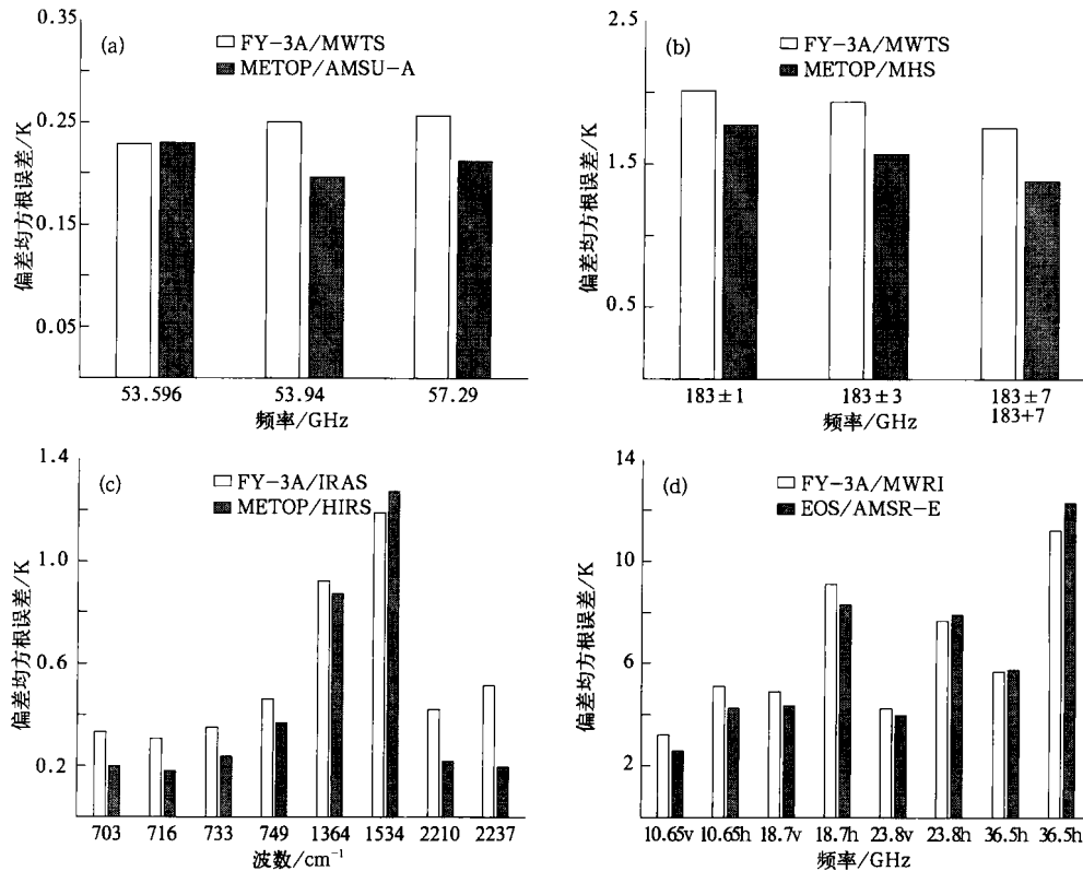
图 4 同化系统中所用 FY-3A 资料模拟偏差均方根误差比较(偏差订正后)
